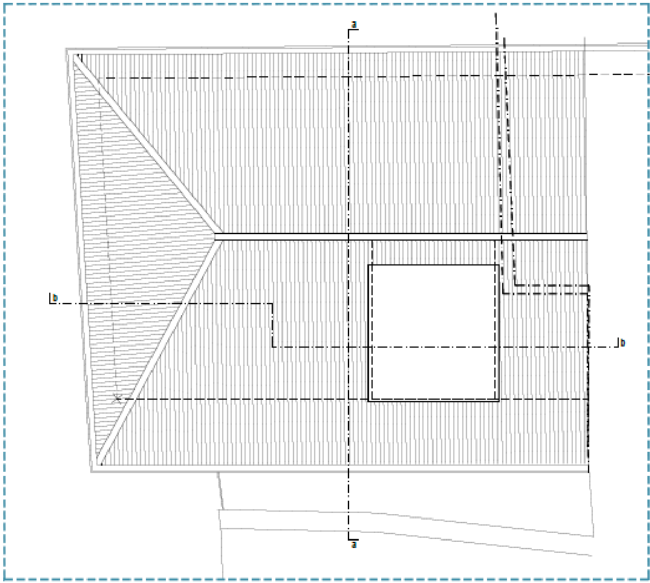
PIANTA COPERTURA - PROGETTO
