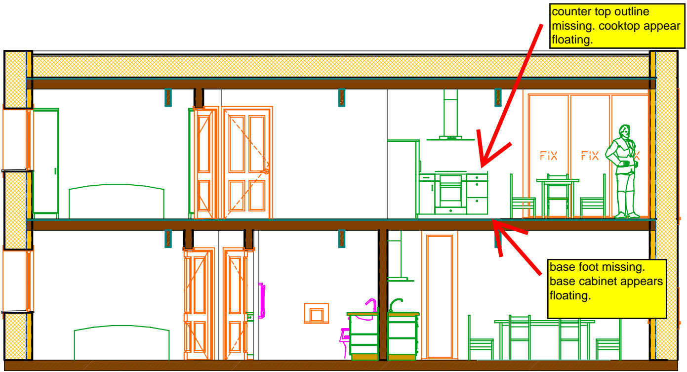
LONGITUDINAL SECTION
