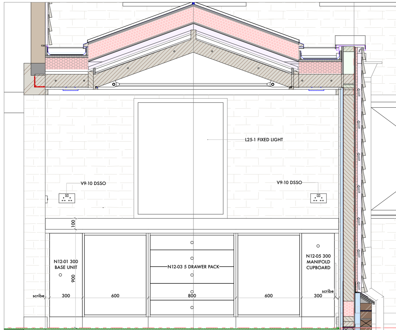
BAR ELEVATION
